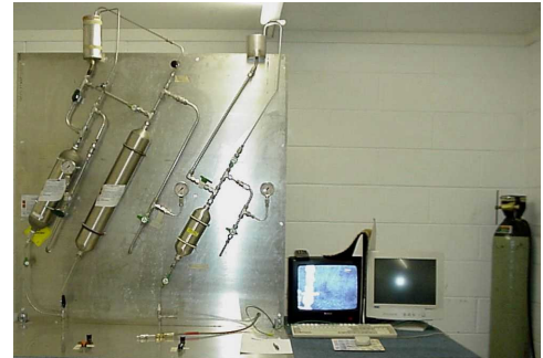
Teststand für den 50%-Antrieb
